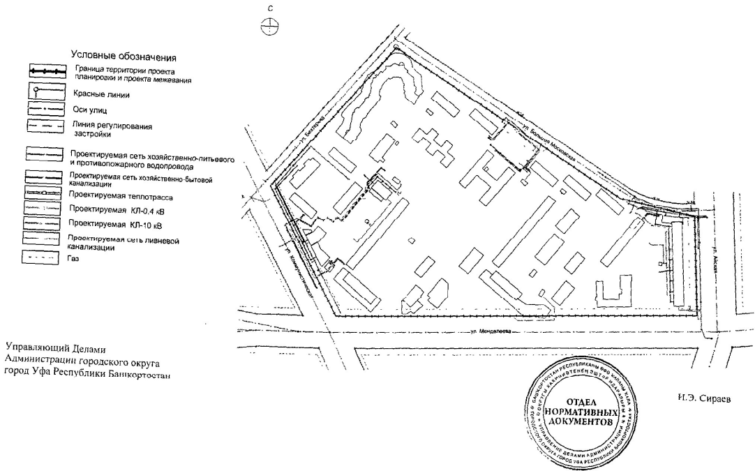
Чертеж планировки территории с отображением красных линий и объектов инженерной инфраструктуры
